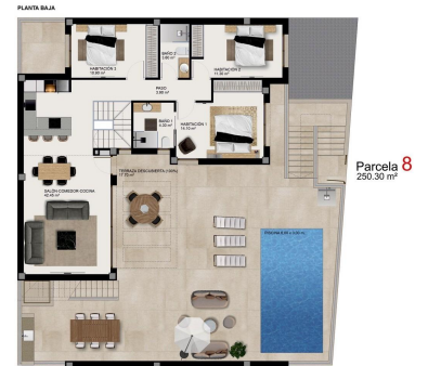
PARCELA 8 Sub. Construido Total 218,10 m 2 Sub. Construido Sótano 100,00 m 2 Sub. Construido Planta Bsp 100,00 m 2 Sub. Construido Terraza 17,70 m 2
