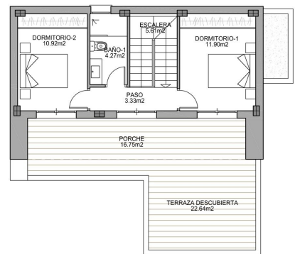
PLANTA PRIMERA
