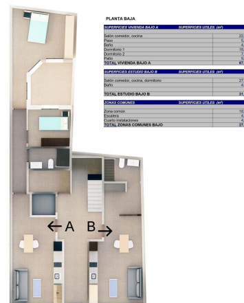
Planta Baja. Estudio B y Vivienda A
