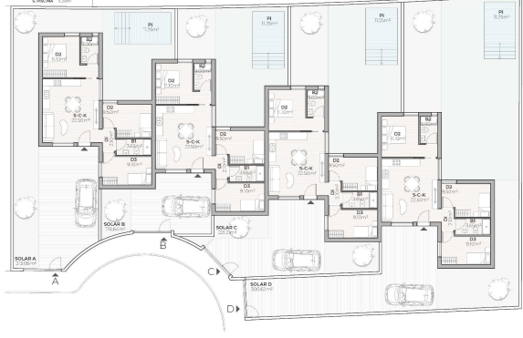
PLANTA BAJA
